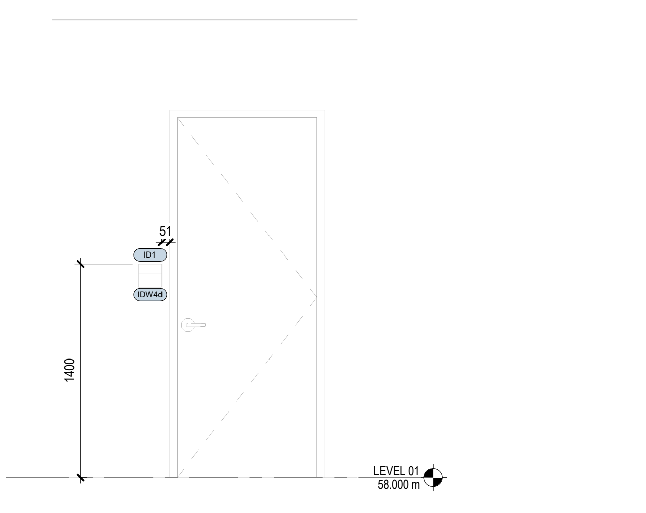
2 TYP. BLADE SIGNAGE- ABOVE DOORS 1:25
